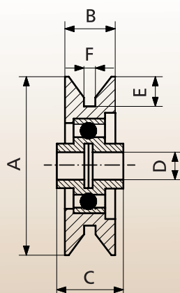
Kladky kovové typ V
